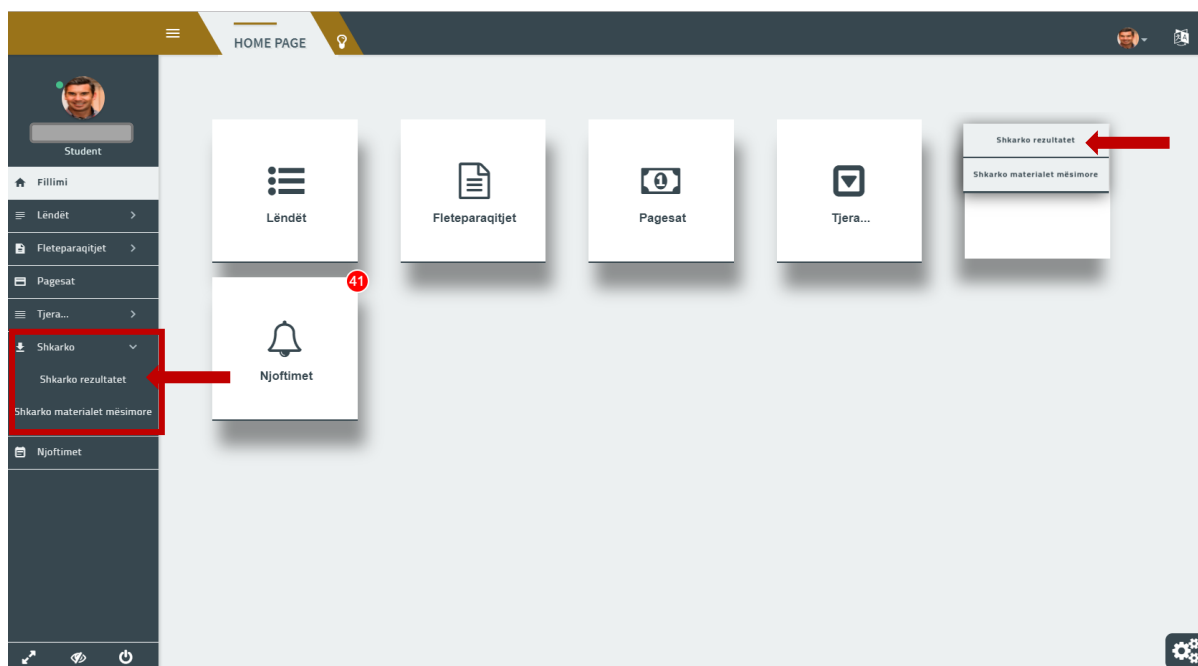
Figure 70:Shkarko rezultatet
